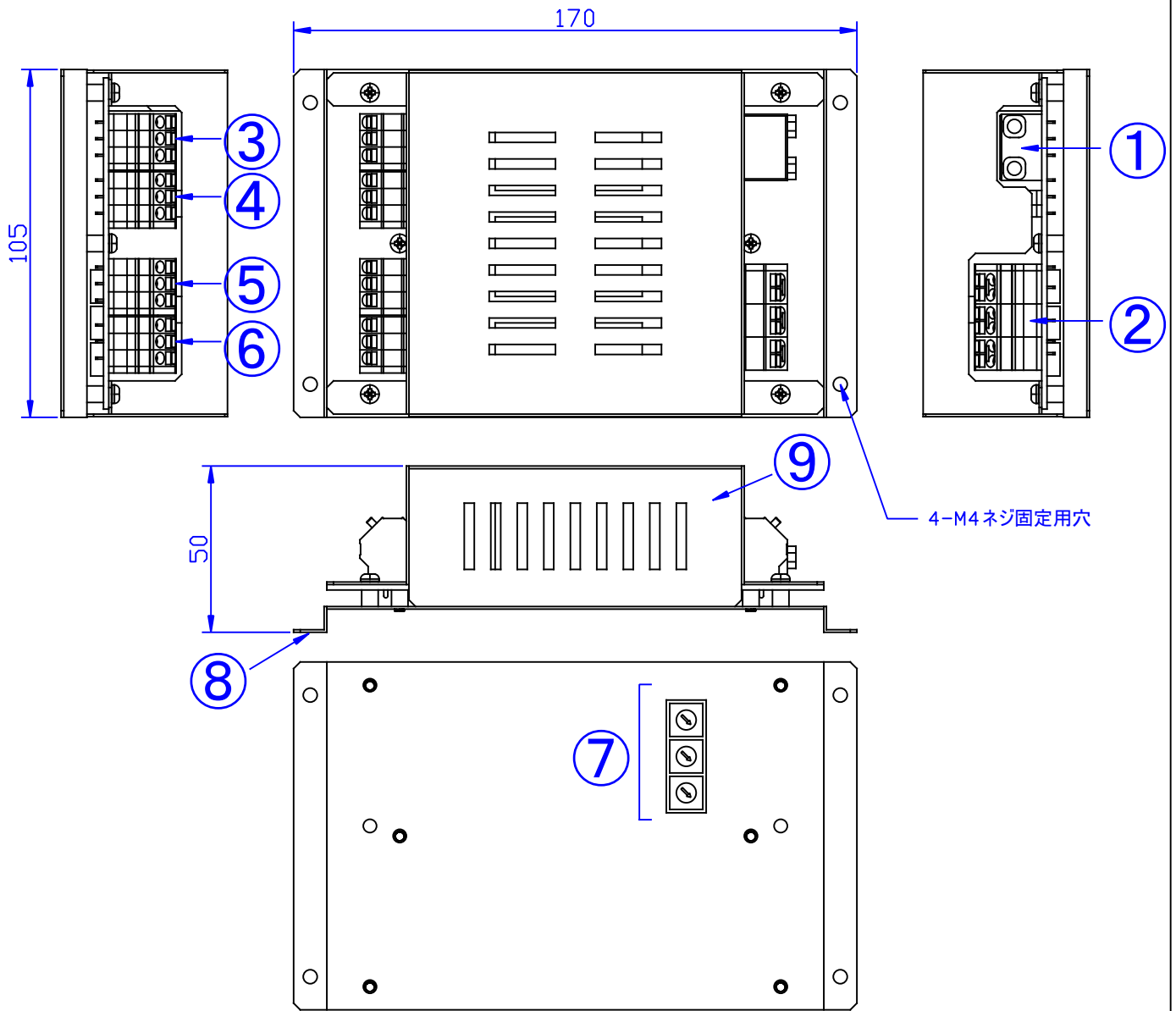
姿図
