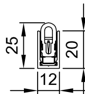
チャンネル取付図 上向き固定時(X-X'断面)(1:1)
