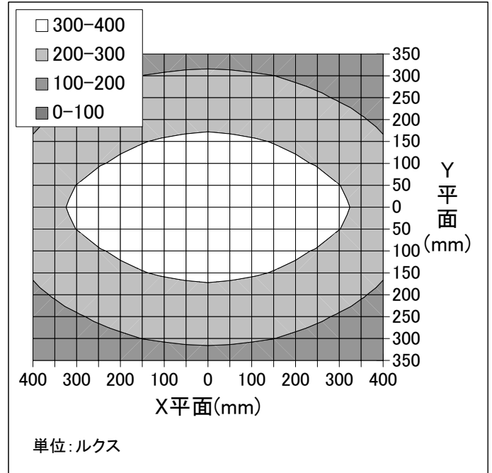
照度分布0.5m直下(昼白色タイプ)
