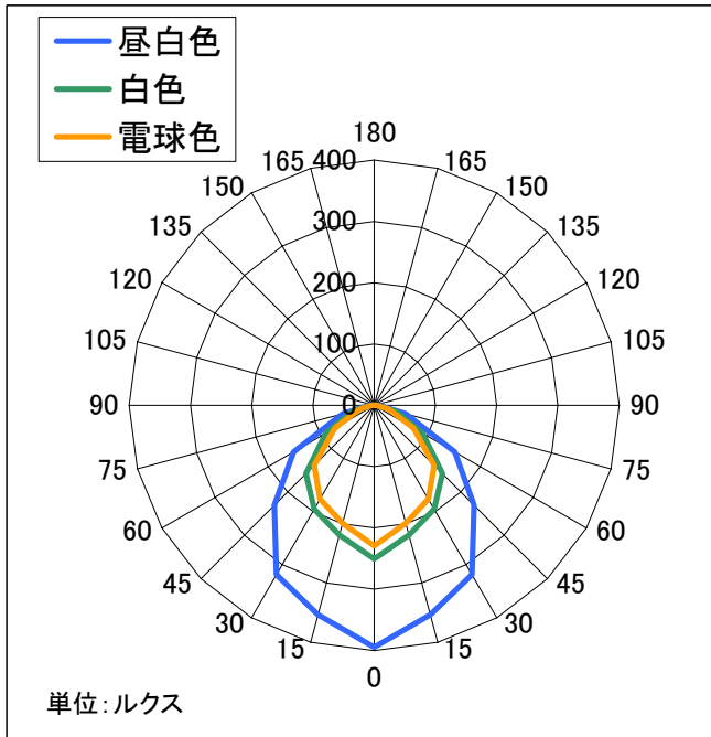
配光曲線0.5m直下
