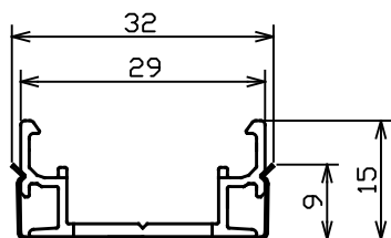
左側面拡大図(1/1)
