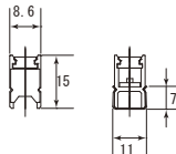
A-A断面図 ホルダー寸法
